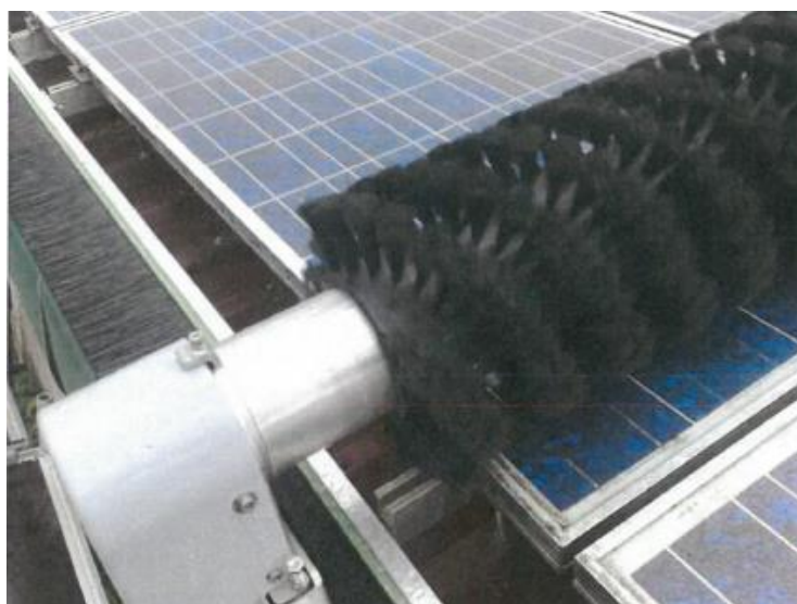
Zdjęcie 6. Szczotka do czyszczenia paneli fotowoltaicznych.
