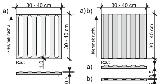
Ryc. 2.7. Płytki kierunkowe do zastosowań: a) na zewnątrz i wewnątrz obiektów, b) do wewnątrz i zadaszonych peronów zewnętrznych. (oprac. autora na podstawie BS 8300, 2000).
