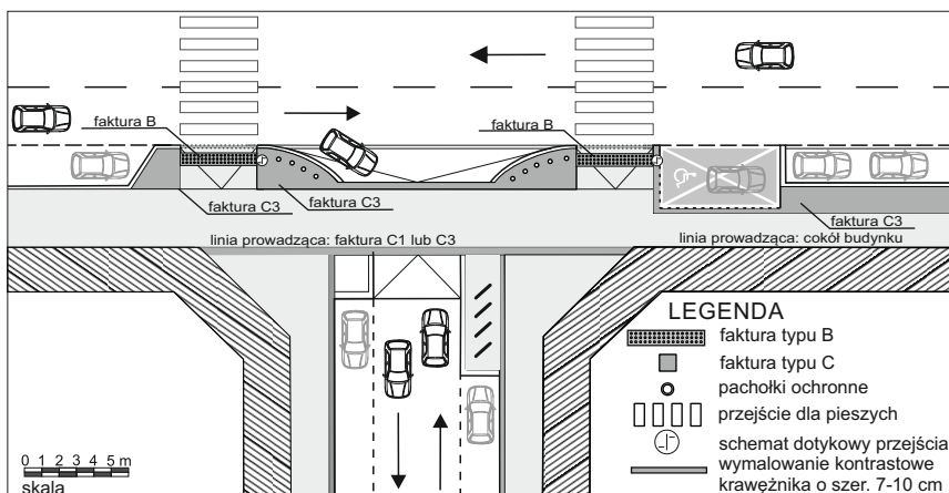
Ryc. 2.4. Przykład zastosowania chodnika przejezdnego na połączeniu z drogą dojazdową lub lokalną lub końcówką białej laski przez osoby niewidome i słabowidzące (źródło: Wysocki 2010, s. 90)
