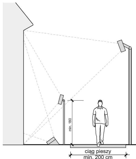
Ryc. 3.6. Lokalizacja opraw oświetlających elewacje budynków. (oprac. autora).
