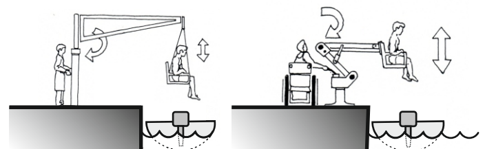
Ryc. 9.12. Przykładowe podnośniki do transportu osób niepełnosprawnych. (oprac. autora na podstawie: X. Ю. Калмет Жилая среда для инвалида 1992, s. 119)
