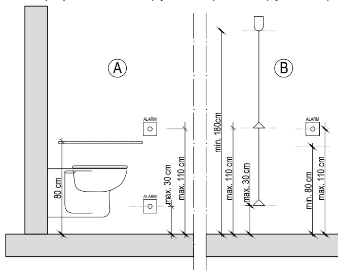
Ryc. 13.6. Schemat montażu przycisków sygnalizacji przywoławczej (oprac. autora)
