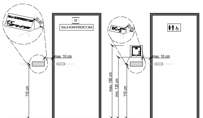
Ryc. 12.7. Miejsce montażu informacji o pomieszczeniu (oprac. autora)
