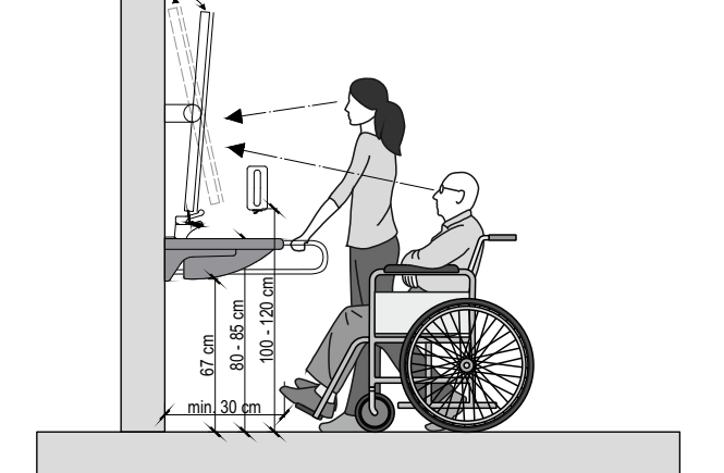
Ryc. 13.4., 13.5. Schemat montażu umywalki, lustra i urządzeń (oprac. autora)
